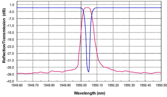
OEDWDM-012 (12.5GHz DWDM FBG)
